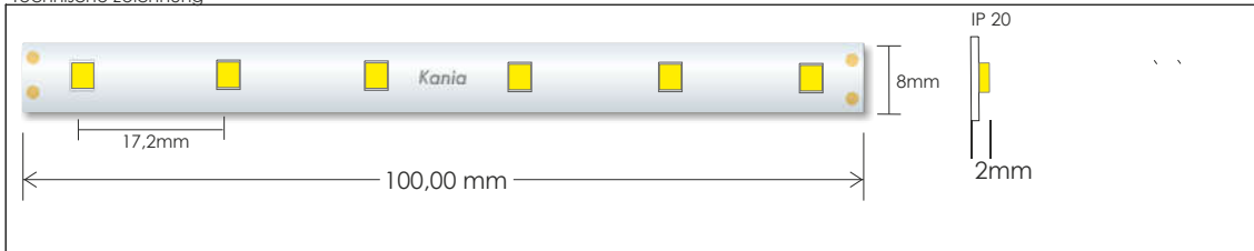
Technische Zeichnung
