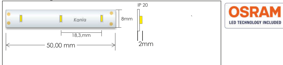
Technische Zeichnung
