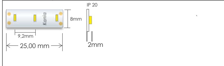
Technische Zeichnung
